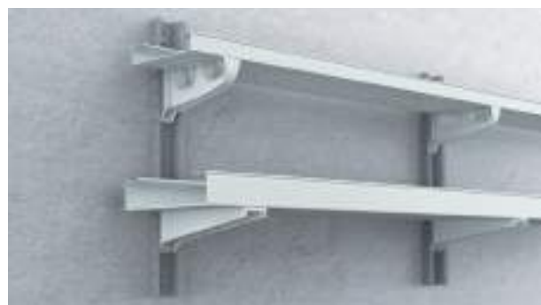
Perfil Omega perforado disponible en: · Acero galvanizado con pintura epoxy gris. · Acero inoxidable AISI 304 con pintura epoxy gris. Con soportes horizontales aislantes en U48X.
